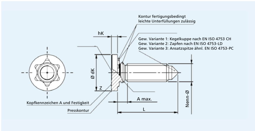
Darstellung Gewindeende: Variante 3
